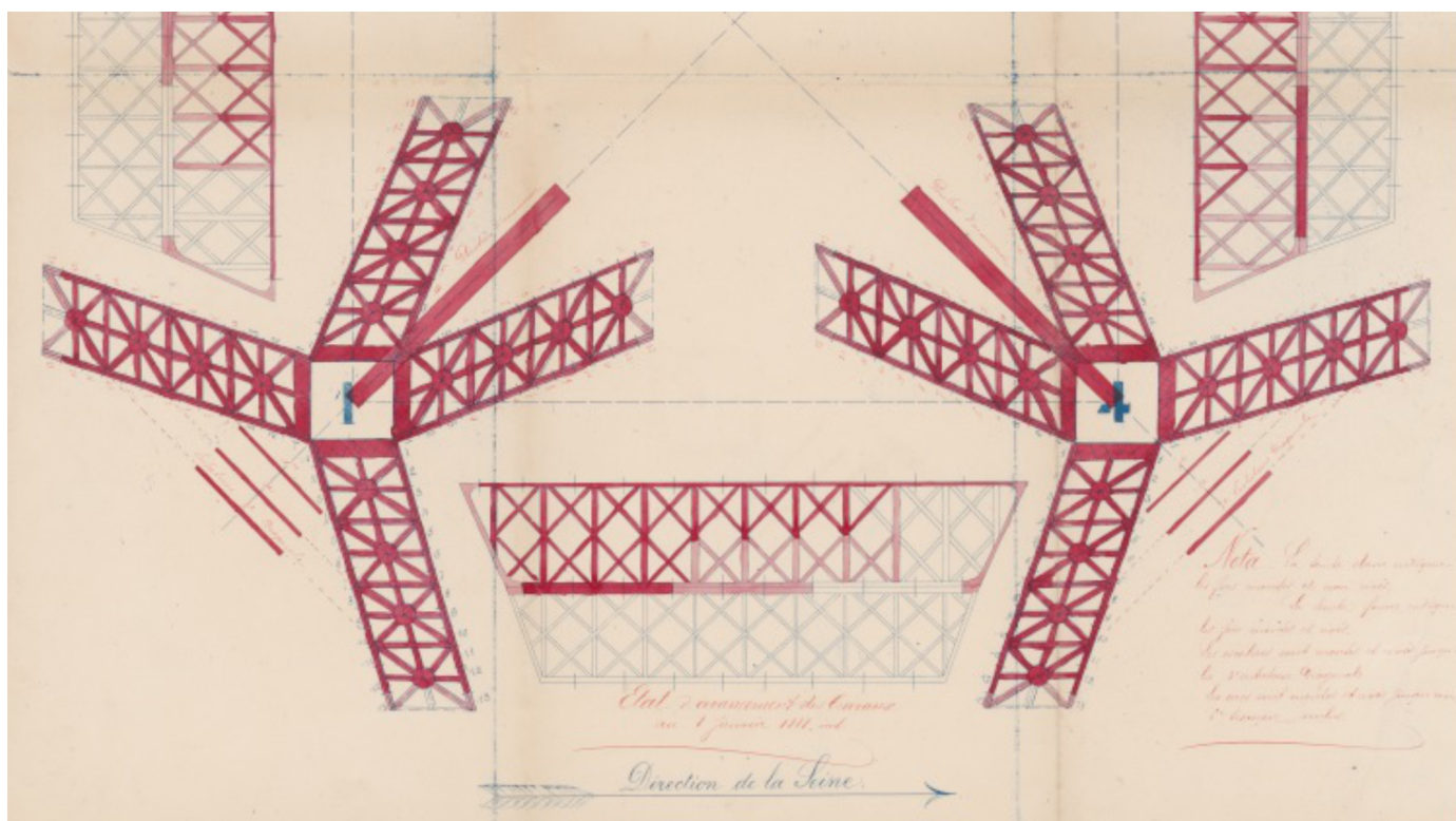
Tour Eiffel, diagramme de montage des ascenseurs, état d'avancement des travaux au 8 janvier 1888, AN : F/12/3871 (Glétaf)
